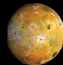
Io
